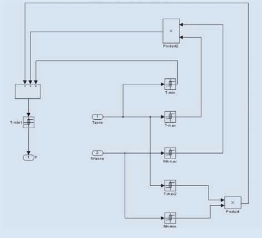
De structuur van een hygrostatiche verwarmingsregelaar in het Simulinkmodel.
