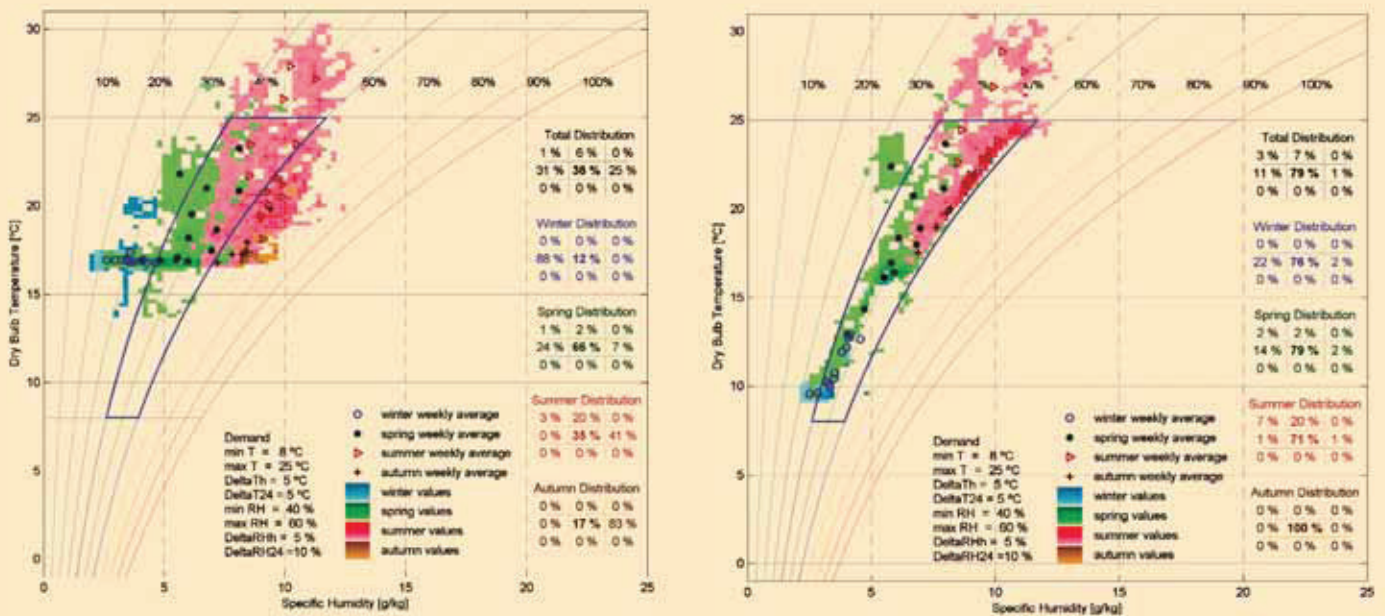
De meetresultaten van de thermostatisch (links) en hygrostatisch (rechts) geregelde vertrekken over de periode van 1 januari tot 1 november 2006. De RV in het hygrostatisch geregelde vertrek ligt voor 14 % van de gemeten waarden onder de 40 %. Voor het thermostatisch geregelde vertrek ligt 32 % van alle meetwaarden onder de 40 %. De RV in het hygrostatisch geregelde vertrek ligt voor slechts 1 % van de gemeten waarden boven de 60 %. Voor het thermostatisch geregelde vertrek geldt dit voor 25 % van alle meetwaarden.
